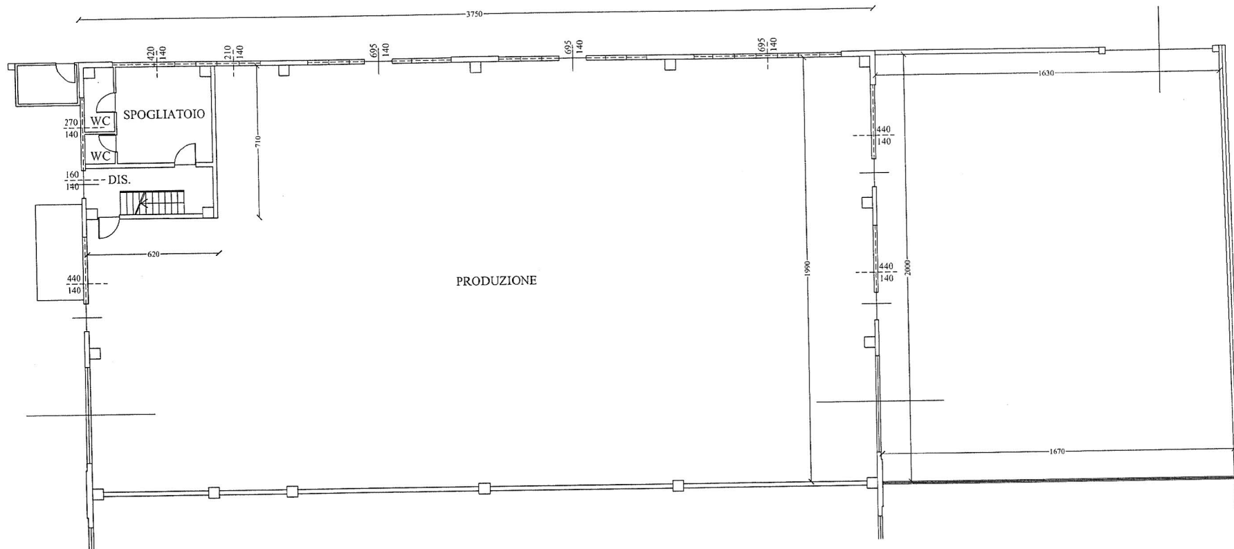
PIANTA PIANO TERRENO
